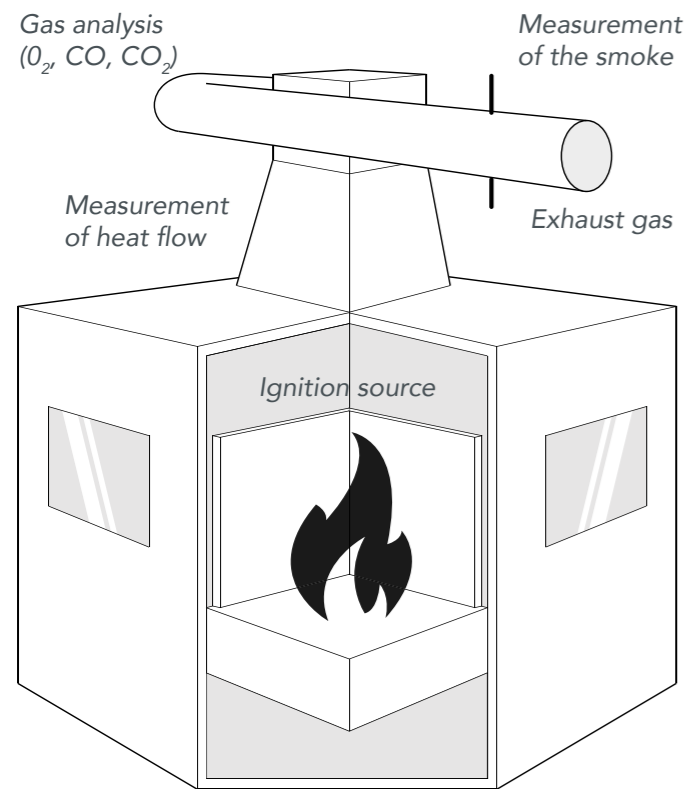
SBI test
